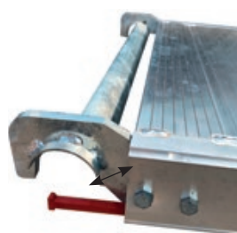
Zuverlässige Abhebesicherung der Platte!
