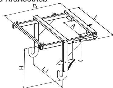
Kippvorrichtung für Stapler- und Kranbetrieb
