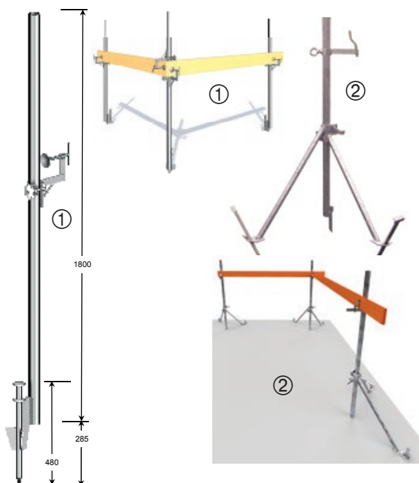
2 Flügel 5/10 cm u. T-Anker abgeschrägt
