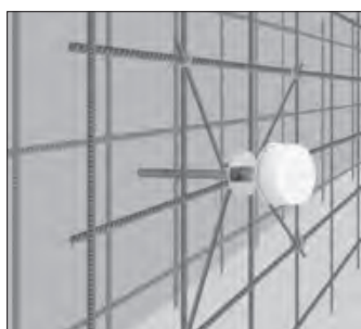
Erdungsfestpunkt mit Bewehrungshalter an der Bewehrung
