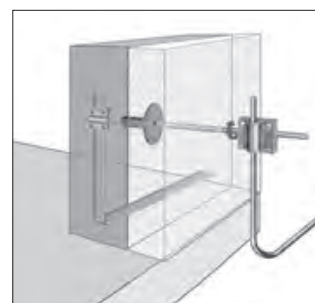
Am Erdungsfestpunkt können sie beidseitig sowohl mit Rund- als auch mit Flachleiter anschließen.
