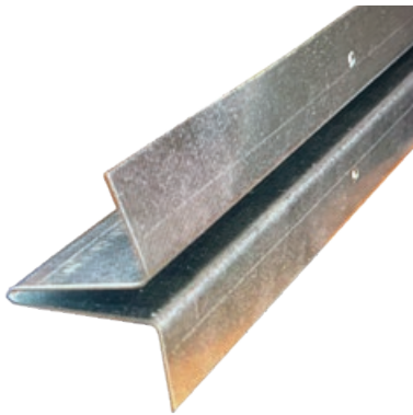
V-Aussparungsprofil für Fugenbleche Wird an die Schalung genagelt und mit der Sole mitbetoniert. Danach wird das Profil entfernt und in die Vertiefung kann das Fugenblech eingeklebt werden. Das Profil kann wieder verwendet werden.
