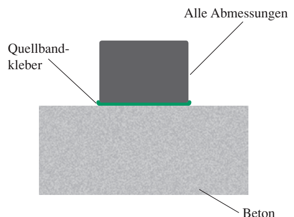
Mit Quellbandkleber
