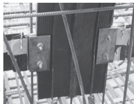
Dichtblech- Fugenbandanschluss
