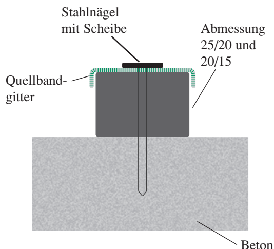
Mit Quellbandgitter
