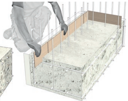
Zurechtbiegen, einstecken und dann mit Haltespange sichern.
