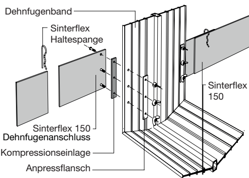
Übergang, Fugenbandanschluß - VIBA-Sinterflex
