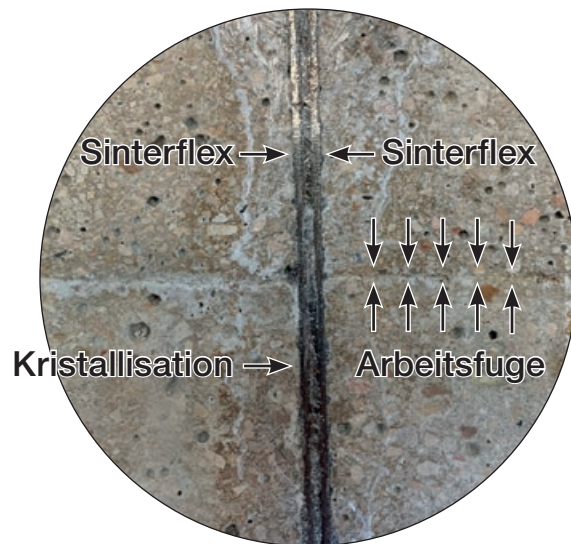
Sinterflex im Stoßbereich
