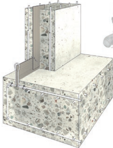
V-Aussparungsprofil für Fugenbleche Wird an die Schalung genagelt und mit der Sole mitbetoniert. Danach wird das Profil entfernt und in die Vertiefung kann das Fugenblech eingeklebt werden. Das Profil kann wieder verwendet werden.
